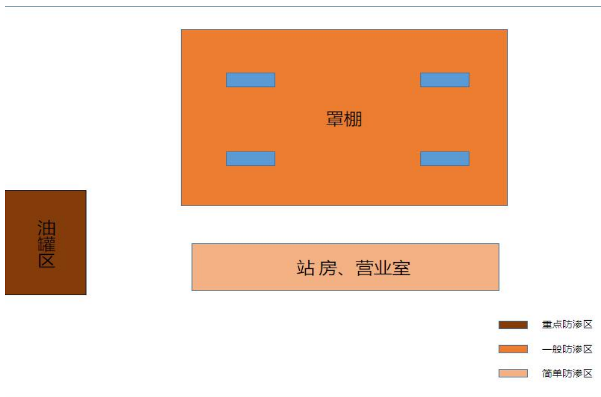
加油站分区防渗图:
