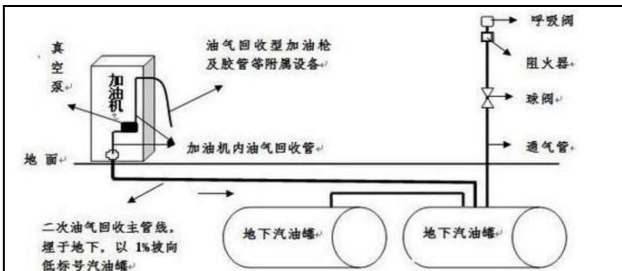
图 5-3 二次油气回收系统基本原理图
