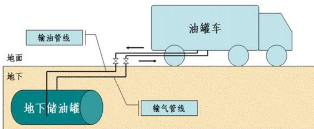
图5-2 一次油气回收系统基本原理图
