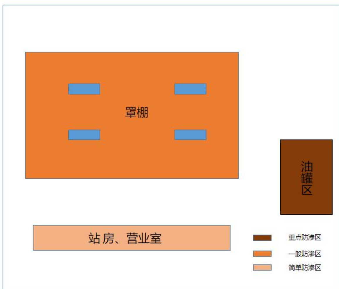
加油站分区防渗图：
