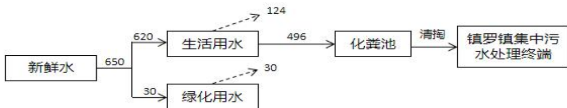
图 1-1 项目水平衡图 单位: \text{m}^3/\text{a}
