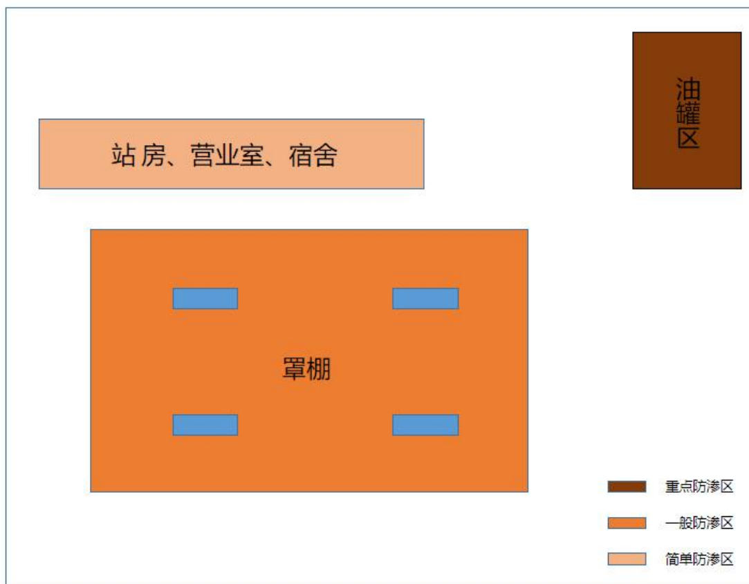
加油站分区防渗图：
