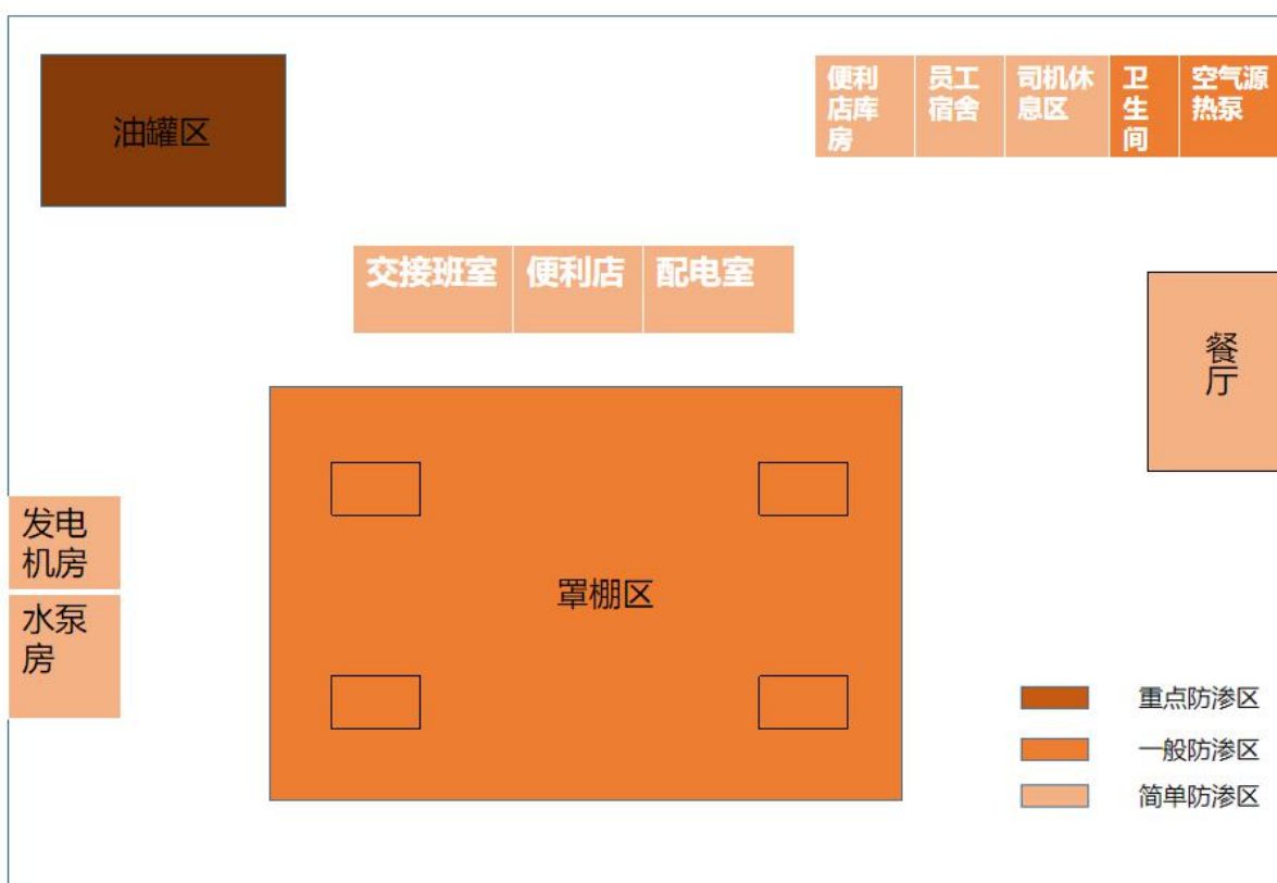
加油站分区防渗图
