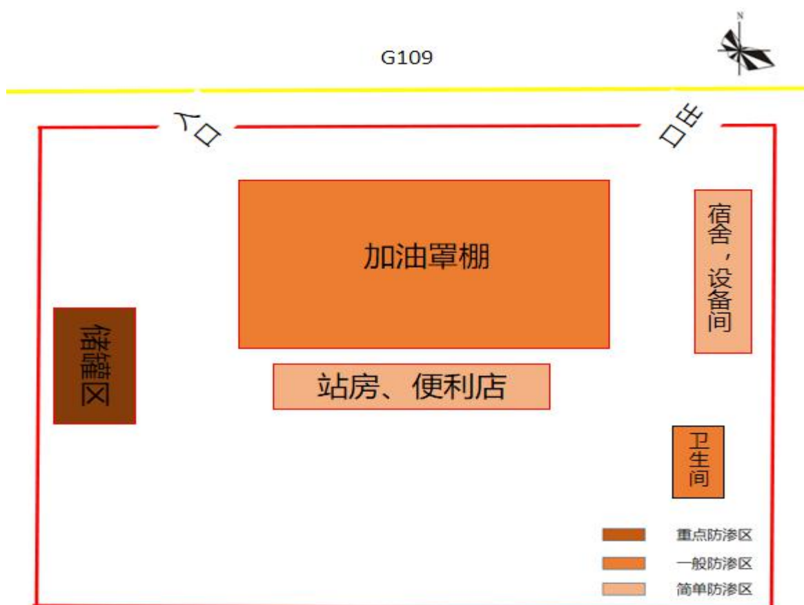
加油站分区防渗图
