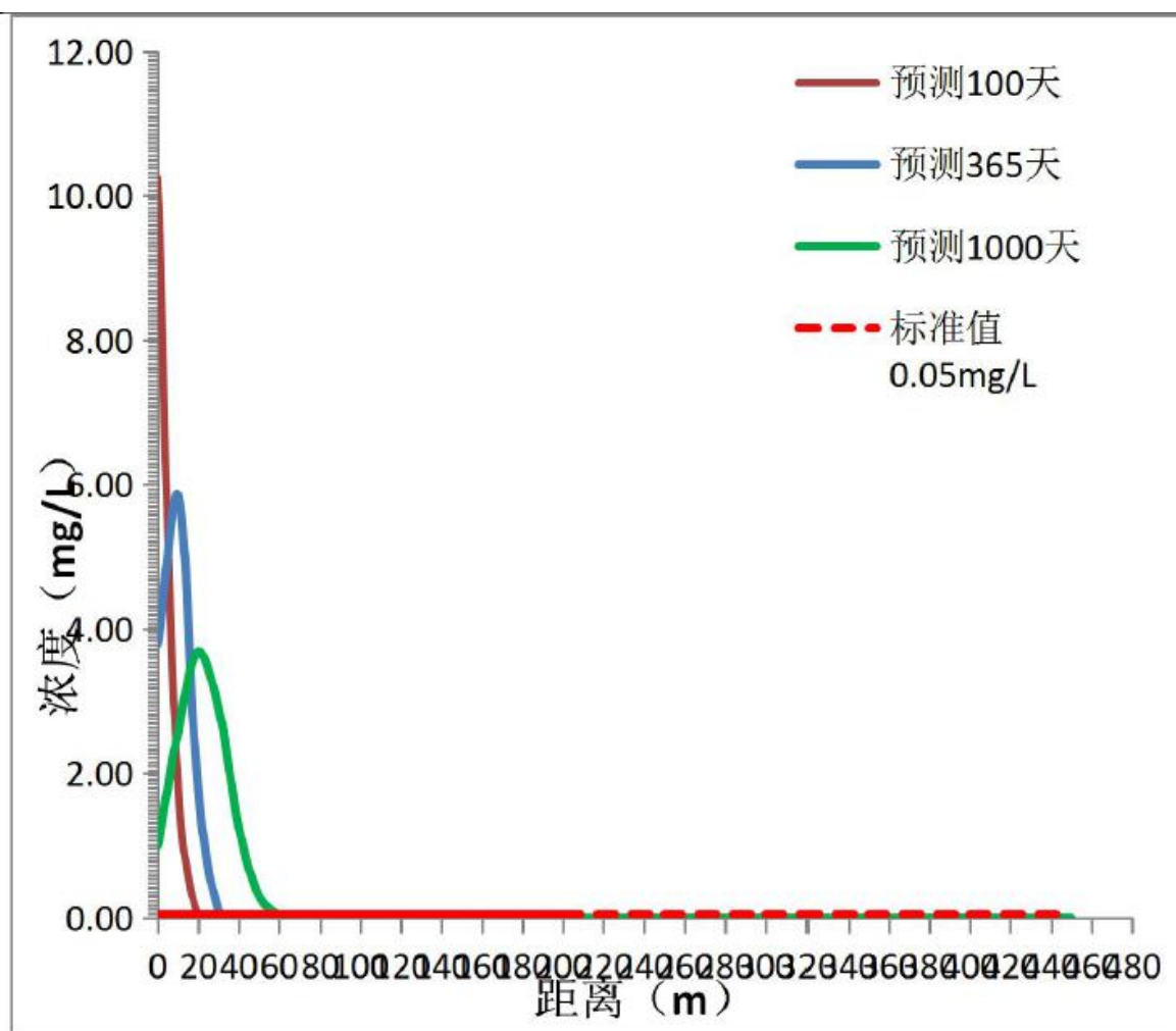
图 7-1 石油类泄漏后随距离、时间衰减的浓度贡献图
