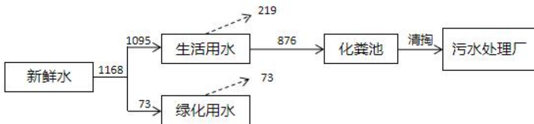
图 1-1 项目水平衡图 单位：m 3 /a
