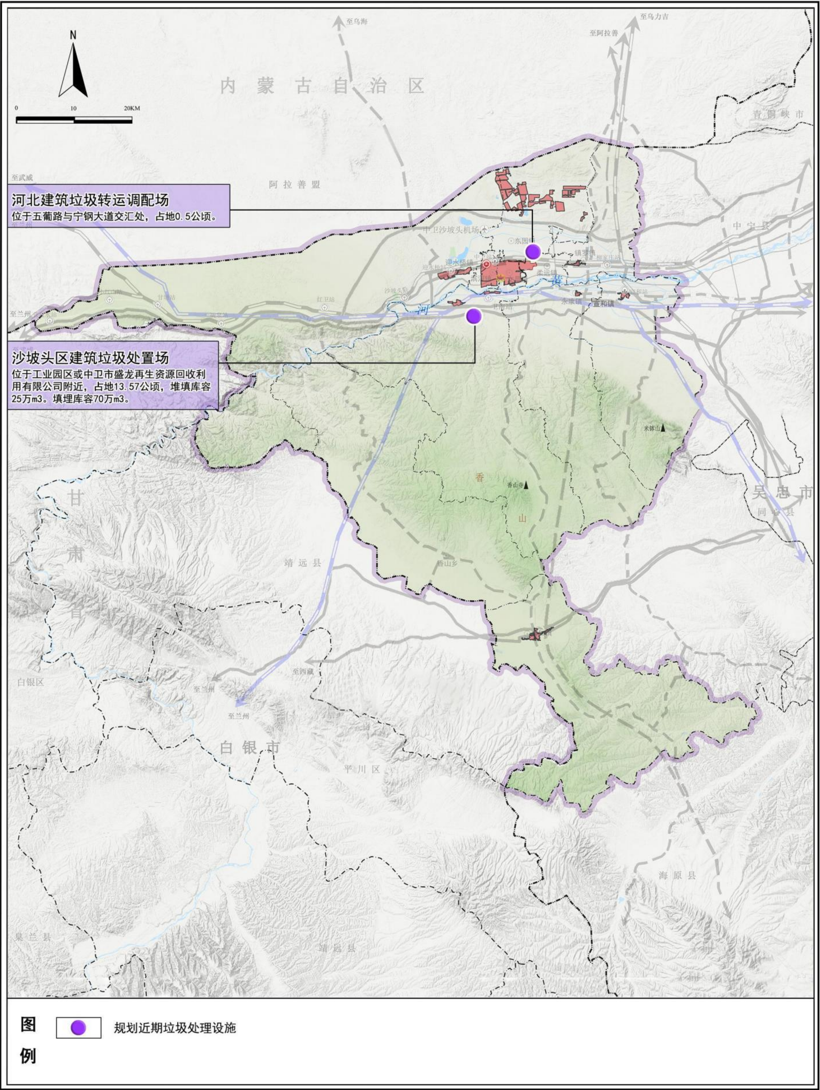
附图四 近期建筑垃圾处置设施规划图
