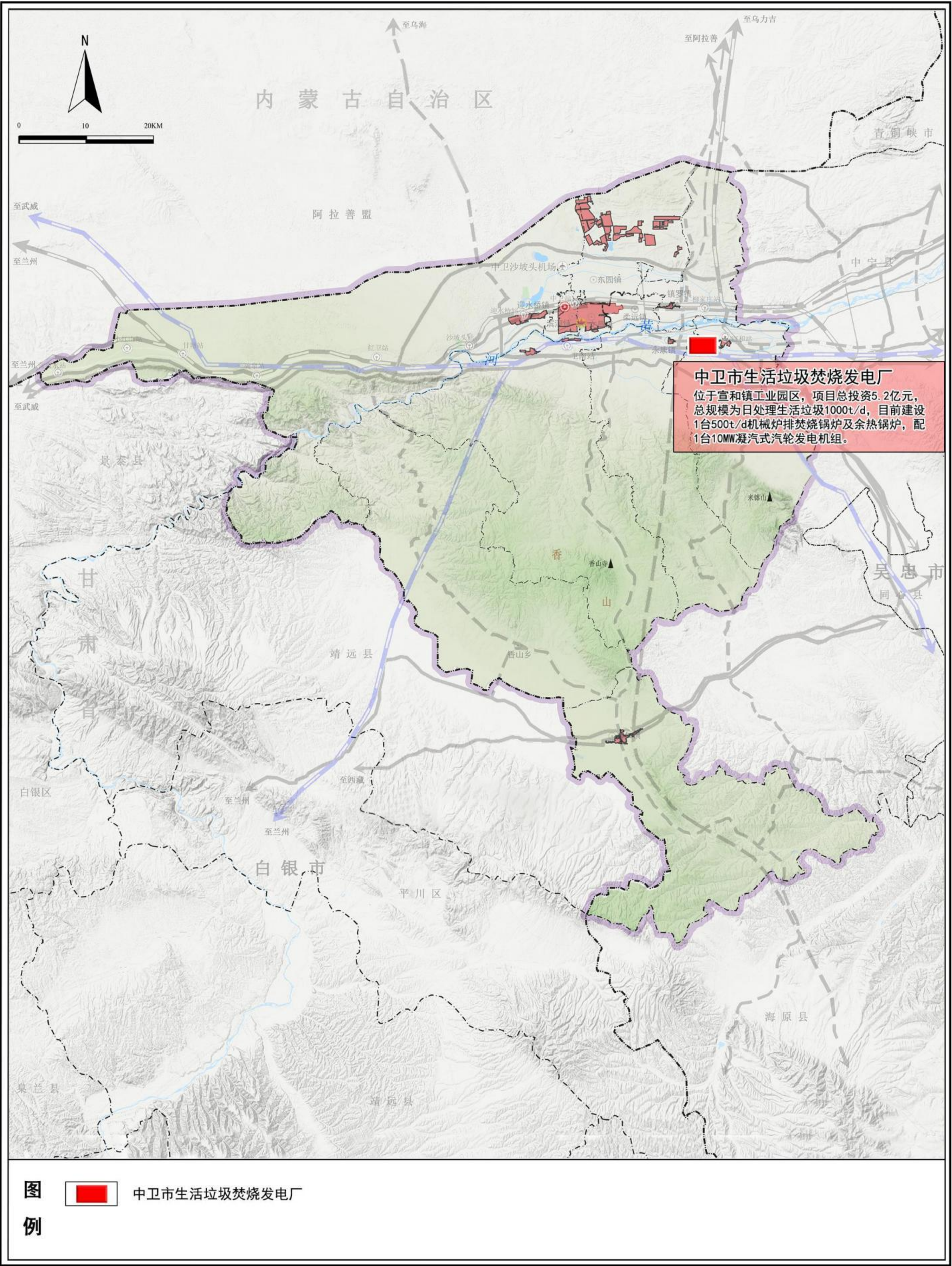
附图六 建筑垃圾分选后可燃物处置规划图
